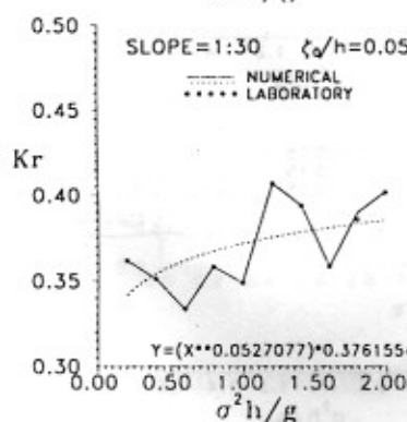
圖5 \zeta_0/h = 0.05 之反射率變化
