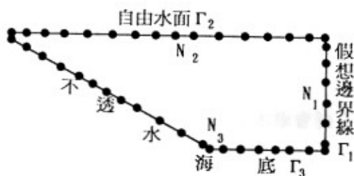
圖 3 數值解析領域定義圖
