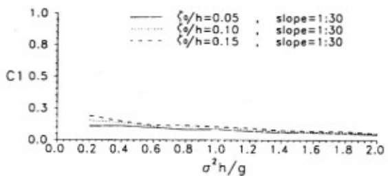
圖 11 C_1 與無因次角週頻率關係圖 (同 Slope)
