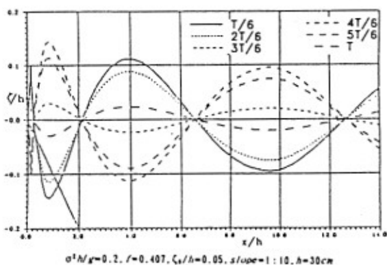
圖 2 \mu = 0 時之波形分佈圖
