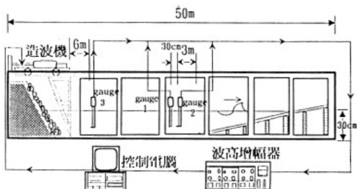
圖 4 實驗場地佈置圖
