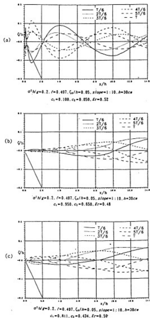
圖8 不同 C_1 、 C_2 組合之波高分佈比較圖
