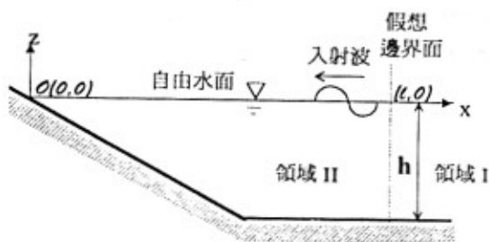
圖 1 岸線斷面地形圖
