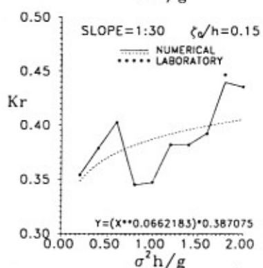
圖7 \zeta_0/h = 0.15 之反射率變化
