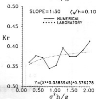
圖6 \zeta_0/h = 0.10 之反射率變化
