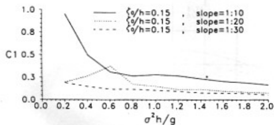
圖 10 C_1 與無因次角週頻率關係圖 (同 \zeta_0/h )
