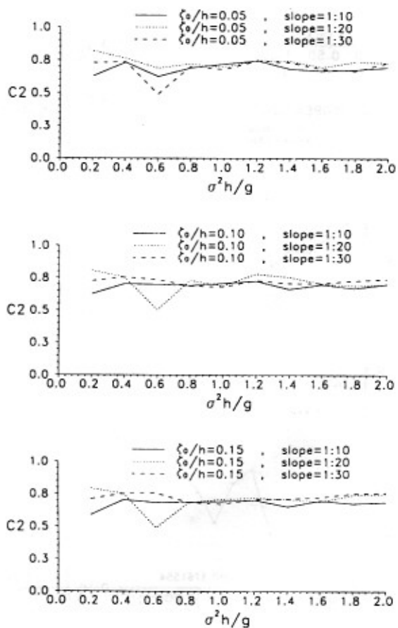
圖9 C_2 與無因次角週頻率關係圖
