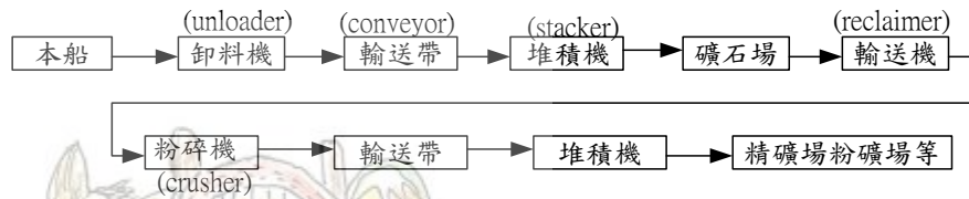
圖 1 礦石類裝卸流程
